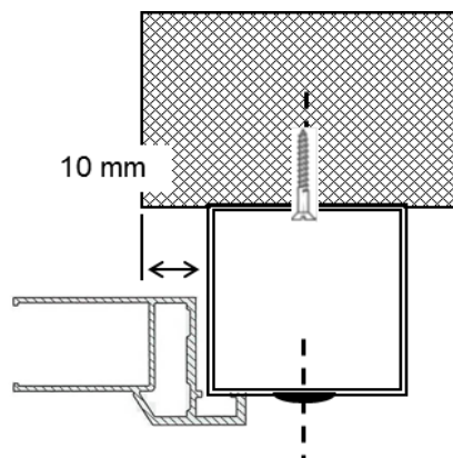
Anschlagprofil (4kt.Rohr) bohren
